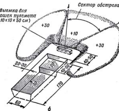
Окопы для стрельбы лежа: а – из автомата; б – из пулемета Окопы для ведения флангового огня должны иметь бруствер со стороны противника высотой 30 см на всю длину окопа
